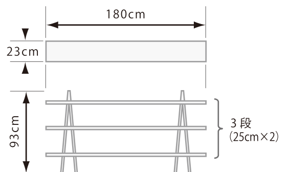
展示棚 (木製)
